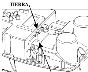
LÍNEA 230Vac-50/60 Hz
